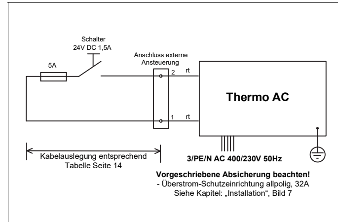
Bild 9: Schaltung mit Schalter, 2-polig
