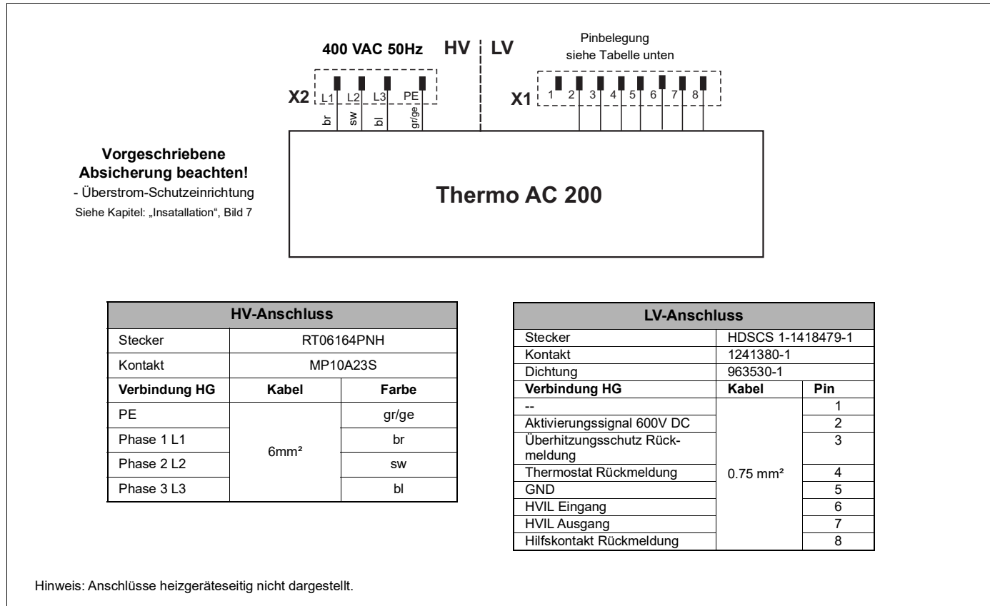
Bild 14: Anschlussplan
