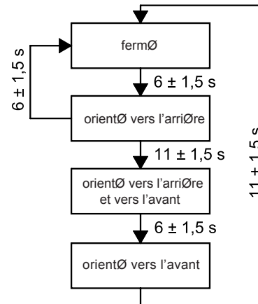
Ill. 302 Déroulement des mouvements avec les durées théoriques
