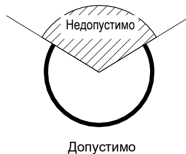
Рис. 806 Позиция сварочного шва камеры сгорания
