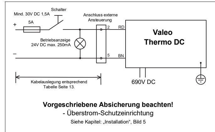
Bild 7: Schaltung mit Schalter, 2-polig, ohne DC/DC Wandler
