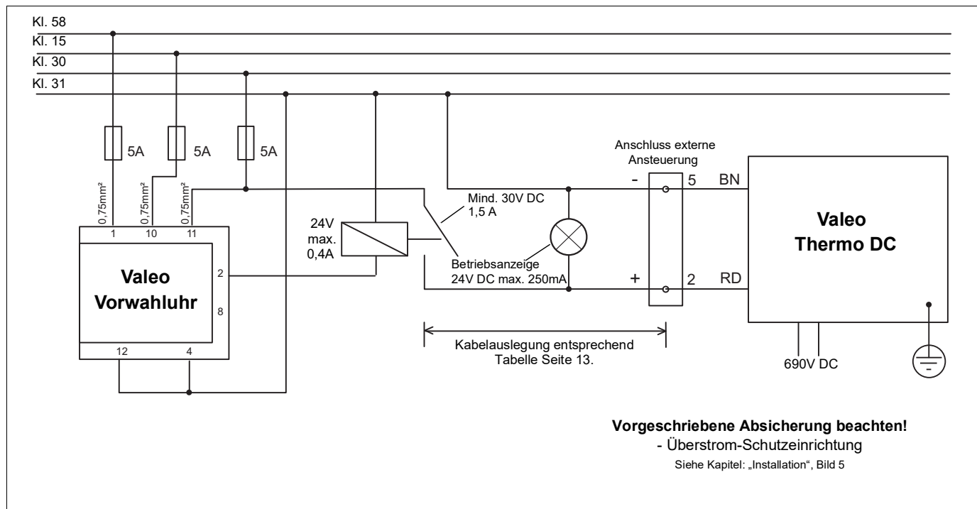
Bild 8: Schaltung mit Vorwahluhr, ohne DC/DC-Wandler
