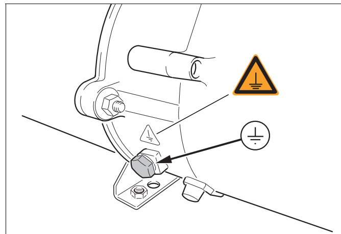
Bild 3: Potentialausgleichsschraube
