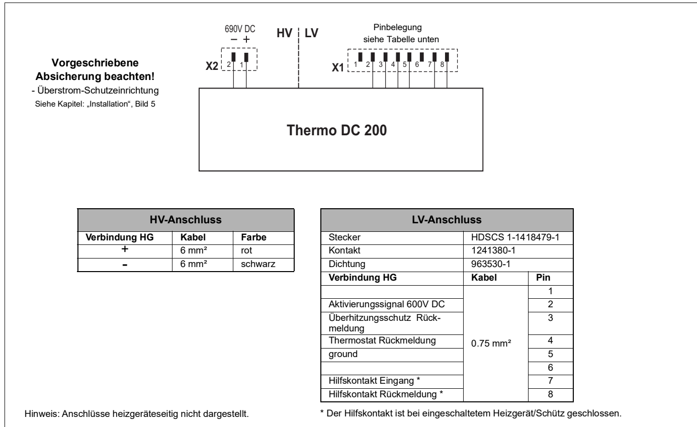
Bild 4: Anschlussplan
