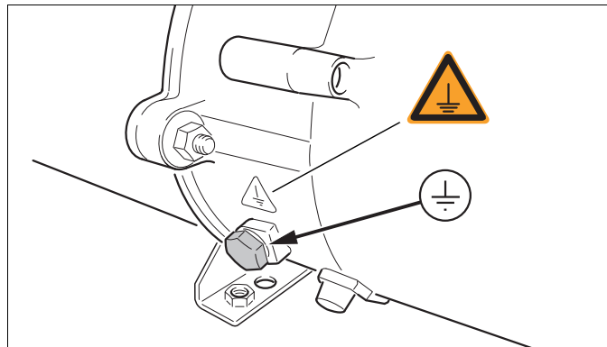
Bild 12: Potentialausgleichsschraube
