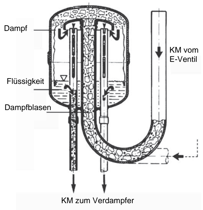
Bild 4-40. Kältemittelverteiler
