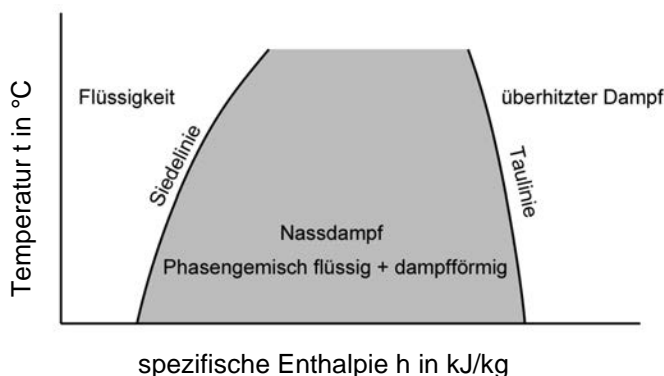
Bild 2-4. t, h-Diagramm
