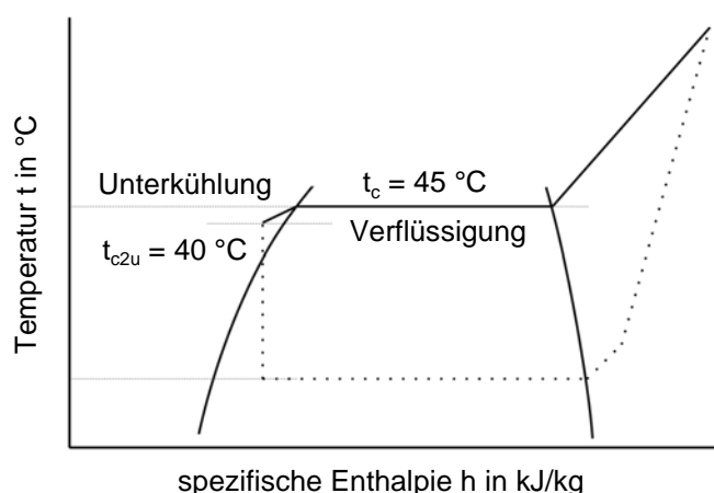
Bild 2-7. Unterkühlung des Kältemittels
