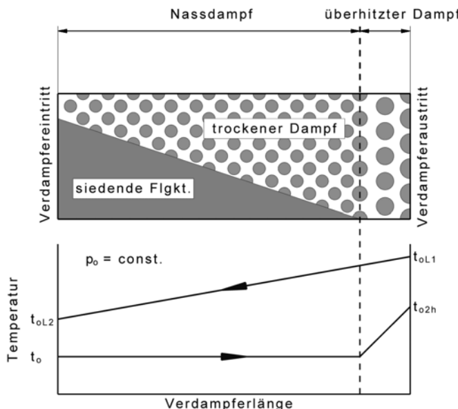
Bild 3-1. Vorgänge im Verdampfer
