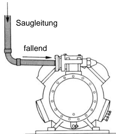
Bild 4-46. Saugleitungsverlegung am Verdichter
