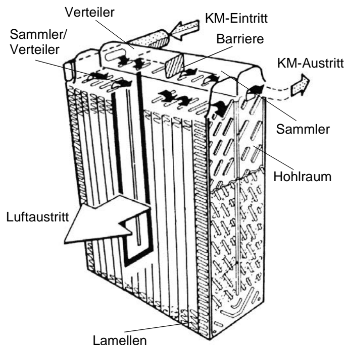
Bild 4-35. Pkw-Plattenverdampfer
