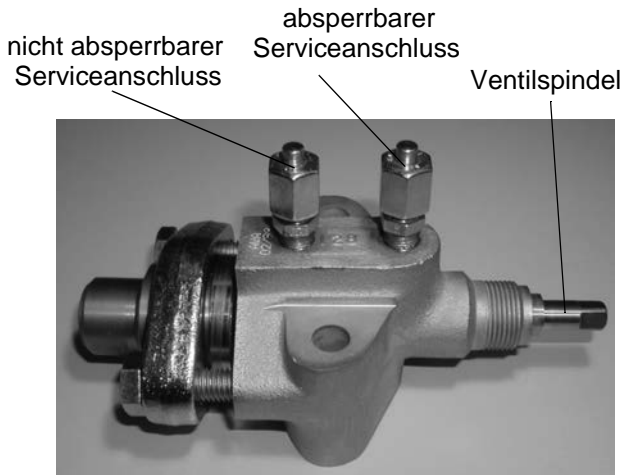
Bild 7-13. Verdichterabsperrventil, Draufsicht
