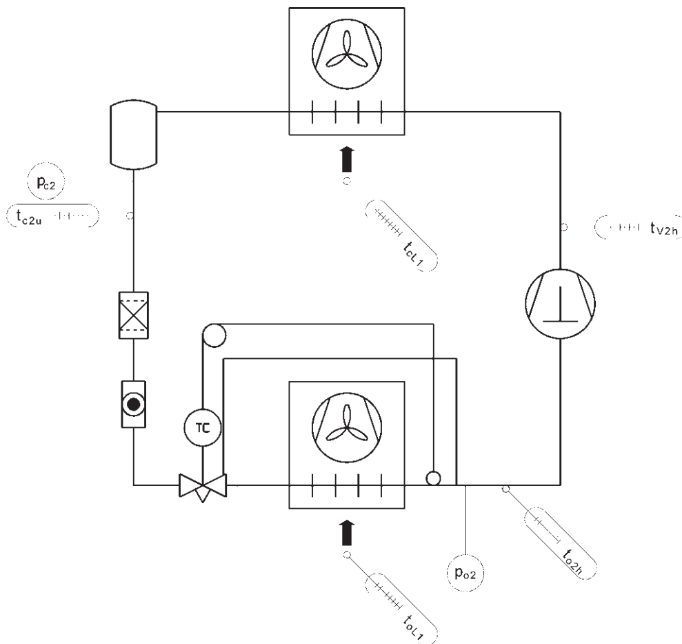
Bild 8-1. Messstellen zur Beurteilung bei der Fehlersuche
