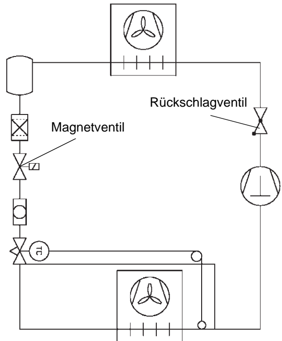
Bild 6-10. Pump-Down-Schaltung
