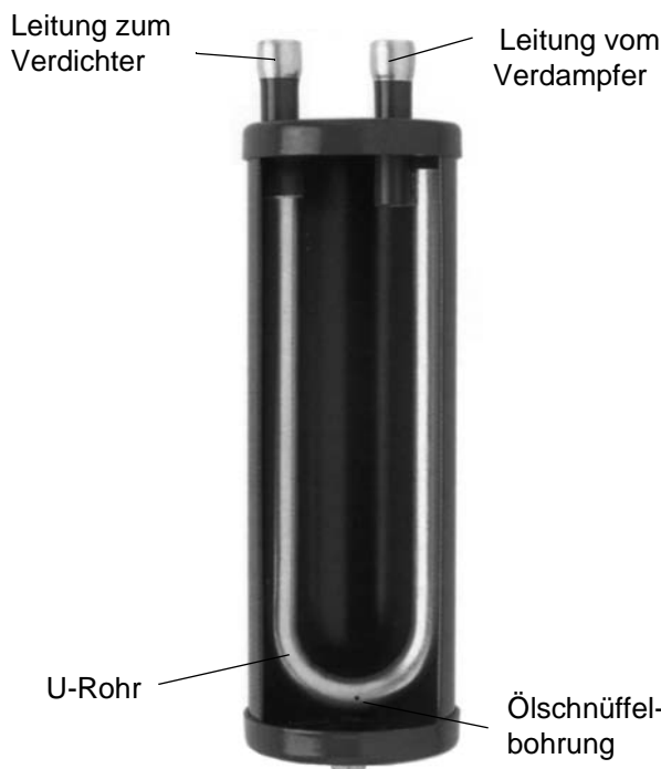
Bild 4-43. Flüssigkeitsabscheider
