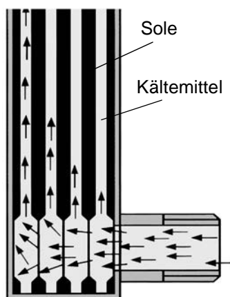
Bild 4-41. Kältemittelverteilung im Plattenverdampfer
