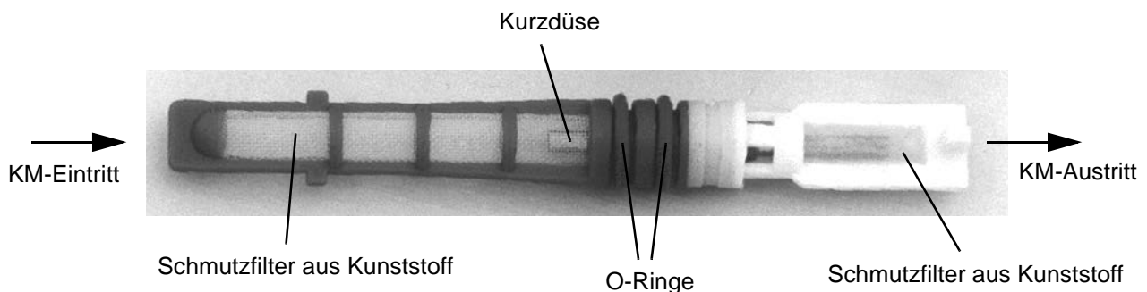
Bild 4-33. Orifice Tube
