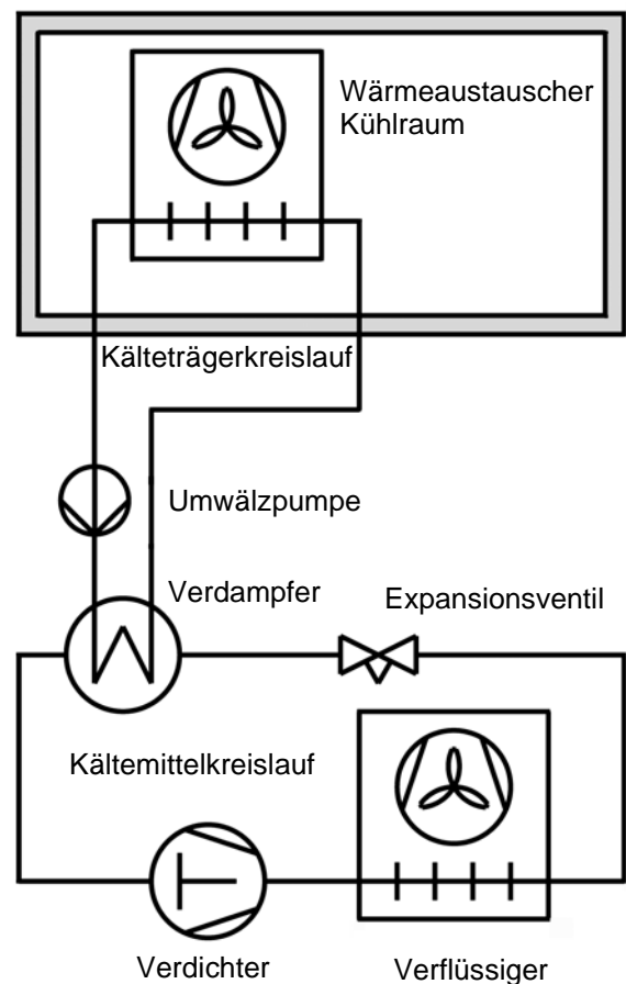
Bild 4-36. Indirekte Kühlung
