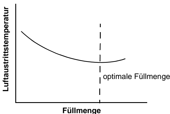
Bild 7-17. Optimale Füllmenge
