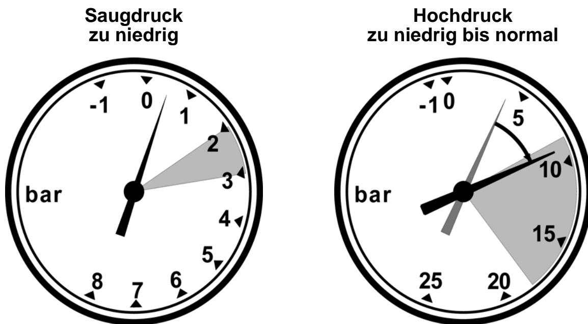
Bild 8-5. Saugdruck zu niedrig, Hochdruck zu niedrig bis normal
