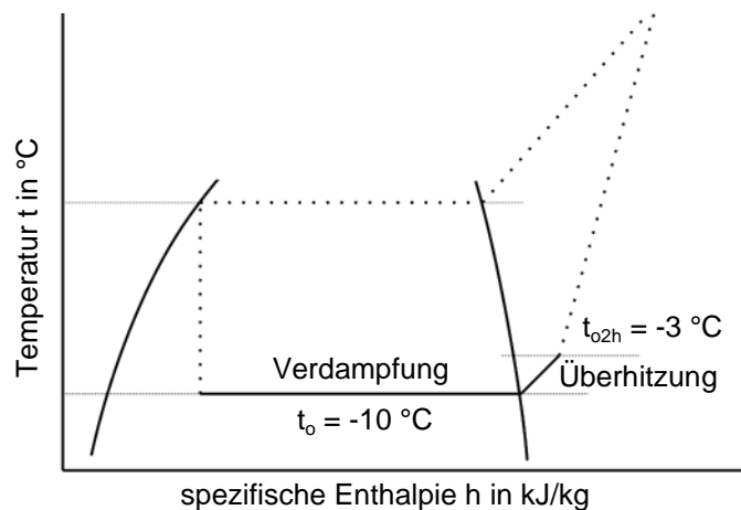
Bild 2-6. Überhitzung des Kältemittels im Verdampfer
