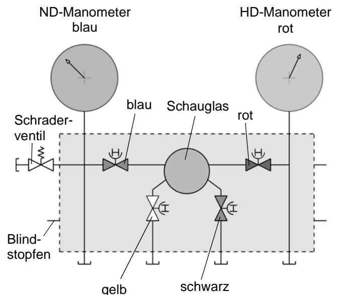
Bild 7-11. Aufbau der Manometerbrücke
