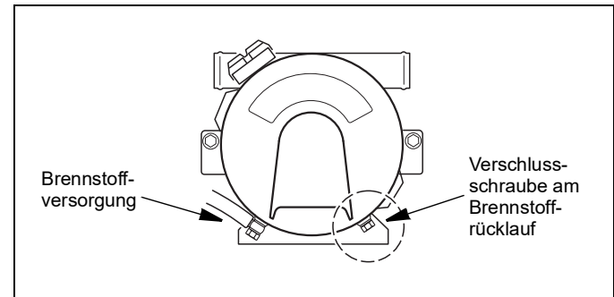
Bild 18: Rücklauf-Verschlusschraube bei Einstrangbetrieb
