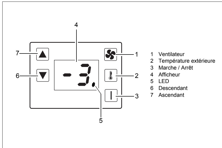
Fig. 1: Commande
