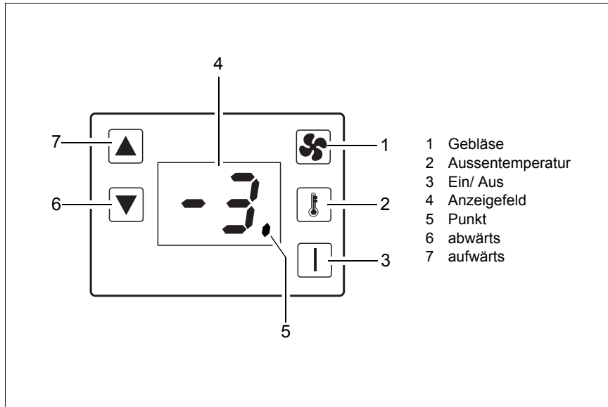
Abb. 1: Bedienteil
