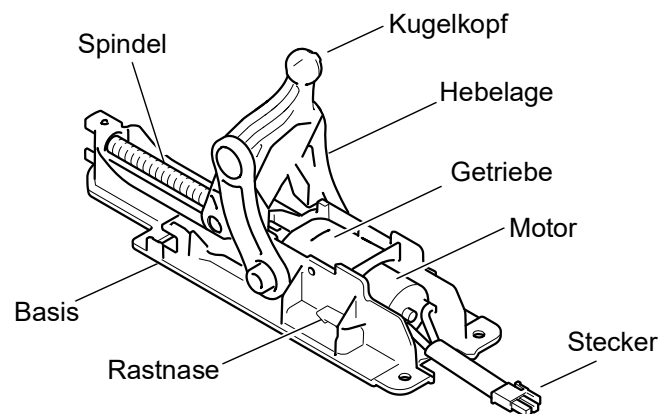
Abb. 302 Ausstellmechanik - elektrisch
