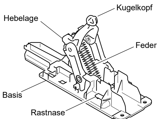
Abb. 301 Ausstellmechanik - manuell
