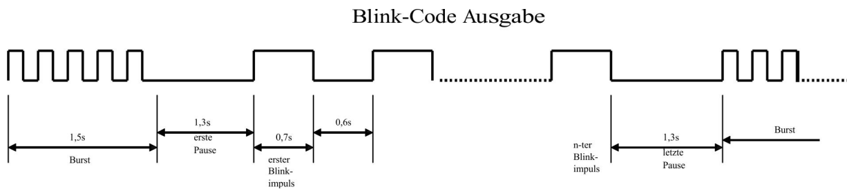
Abb. 401 Blinkcode an der Betriebsanzeige
