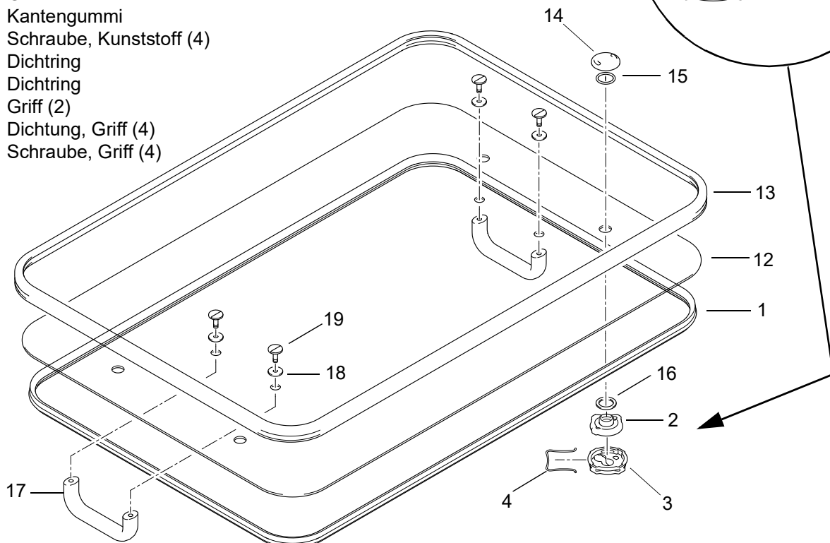
Abb. 304 Eleon Luken - Komponenten (Teil 2)
