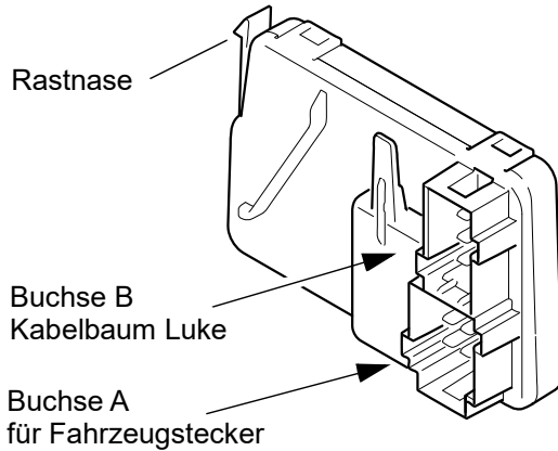
Abb. 305 Steuergerät
