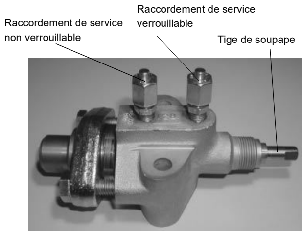
Fig. 7-13 Soupape d'arrêt de compresseur, vue de dessus
