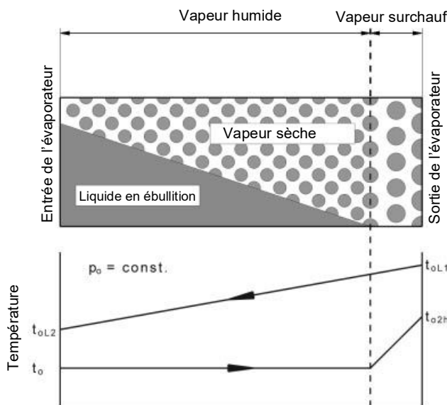
Fig. 3-1. Processus à l'intérieur de l'évaporateur
