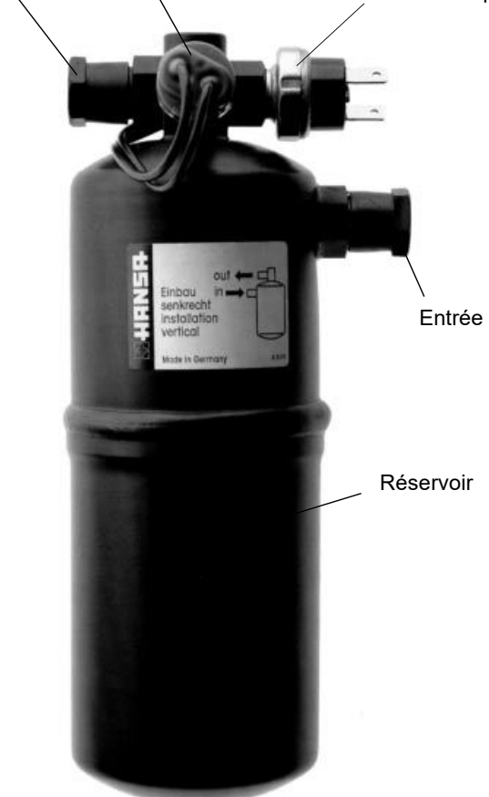
Fig. 4-20. Collecteur d'une installation frigorifique d'automobile
