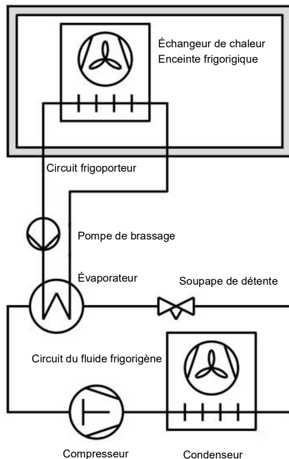
Fig. 4-36. Refroidissement indirect
