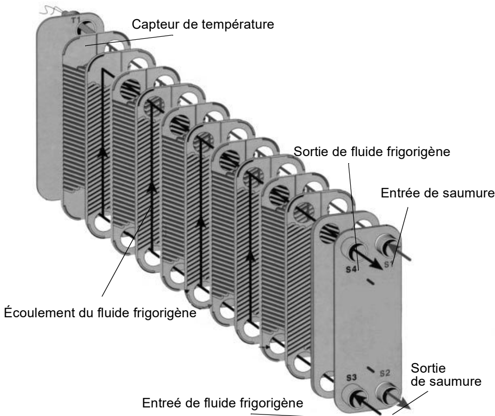
Fig. 4-37. Construction d'un évaporateurs à plaques
