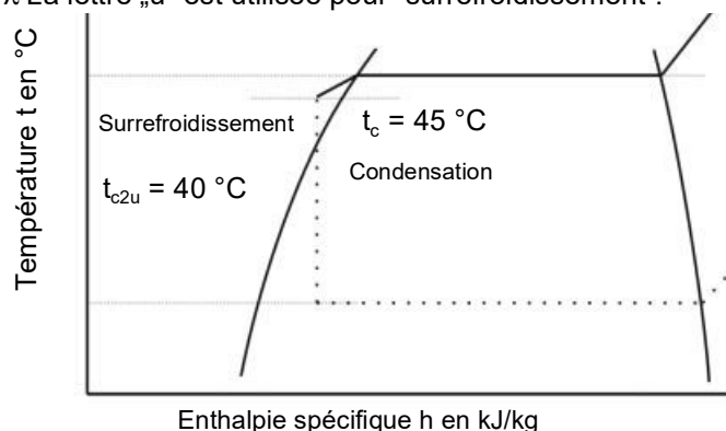
Fig. 2-7. Surrefroidissement du fluide frigorigène
